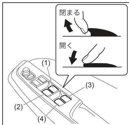
(1) 運転席ウィンドースイッチ (オート機構付)
