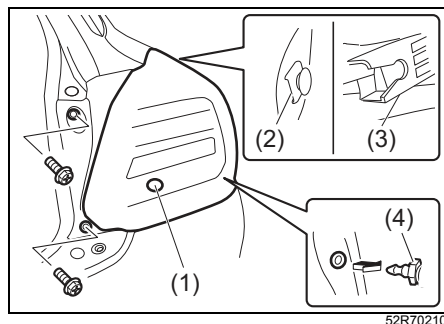
(1) 方向指示器／非常点滅表示灯 (後面、Aタイプ)
